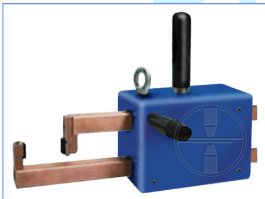
Mikro-C-Hartlötzange Best.-Nr.: XRML.3ZC.001
