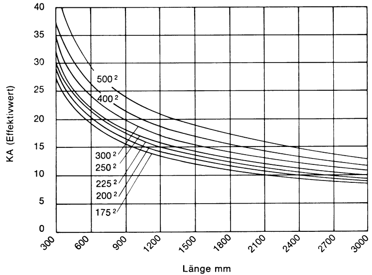
Belastungstabelle für wassergekühlte Schweißkabel (Richtwerte unverbindlich)
